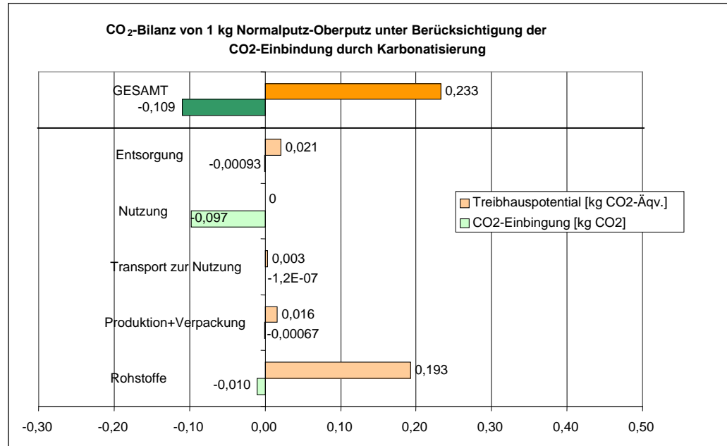
Abbildung 6: CO 2 -Bilanz von 1 kg Normalputz - Oberputz unter Berücksichtigung der CO 2 -Einbindung durch Karbonatisierung
