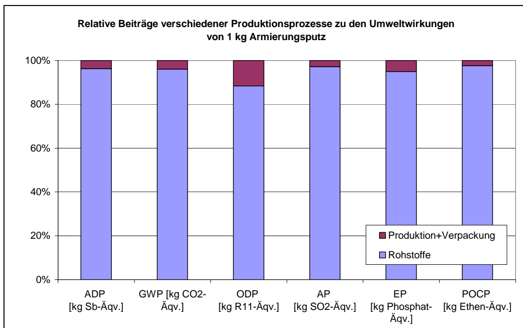
Abbildung 5: Relative Beiträge verschiedener Produktionsprozesse zu den Umweltwirkungen von 1 kg Armierungsputz
