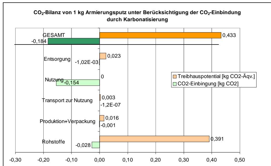
Abbildung 7: CO 2 -Bilanz von 1 kg Armierungsputz unter Berücksichtigung der CO 2 -Einbindung durch Karbonatisierung
