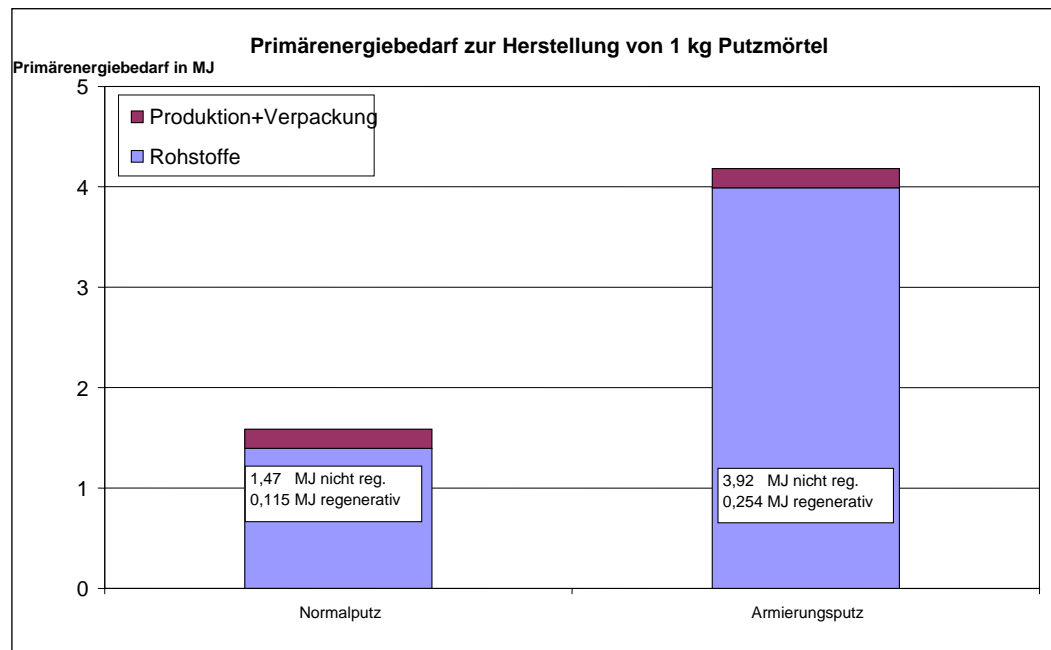
Abbildung 1: Primärenergiebedarf zur Herstellung von 1 kg Putzmörtel
