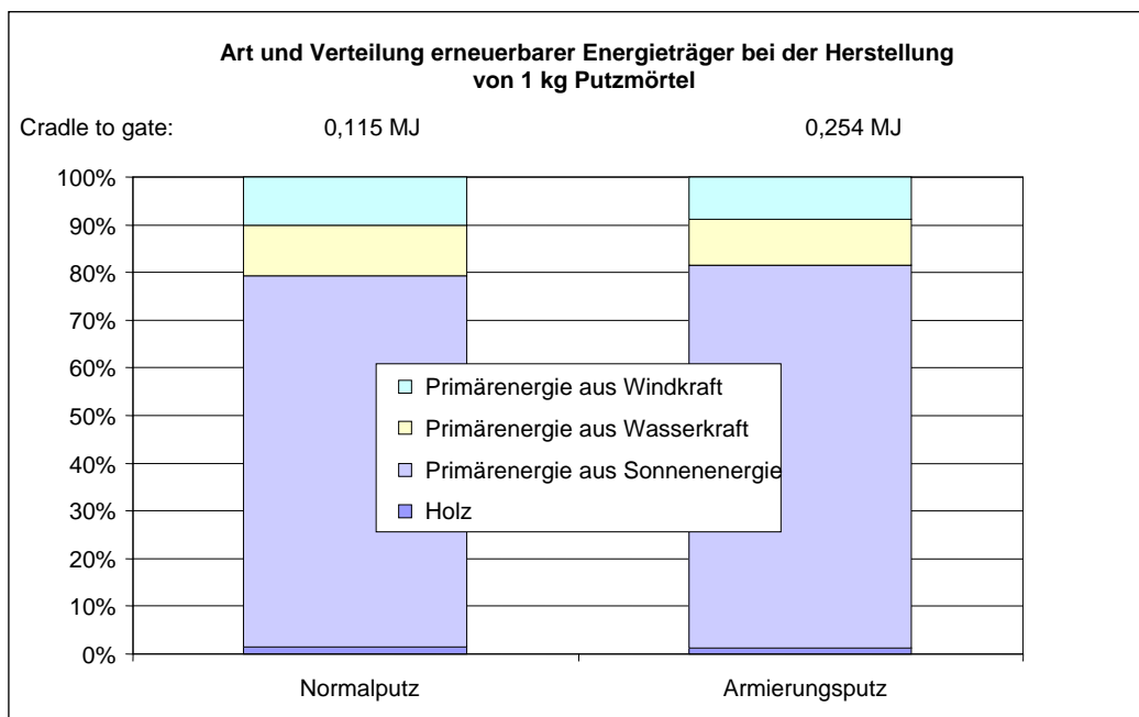
Abbildung 3: Art und Verteilung erneuerbarer Energieträger bei der Herstellung von 1 kg Putzmörtel
